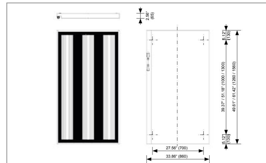
Außen- und Befestigungsmaße der LPS100 PM. Alle Angaben in Inch (mm).
