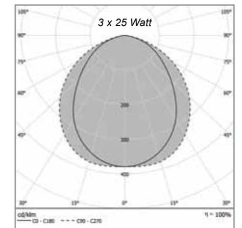
Lichtverteilungskurve der LPS100 PM (LPS100 puremaxLED®). Diese Grafik zeigt die Lichtverteilungskurve einer LPS100 PM mit 3 x 25 Watt
