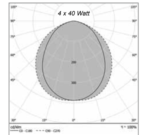
Lichtverteilungskurve der LPS50 PM (LPS50 puremaxLED®). Diese Grafik zeigt die Lichtverteilungskurve einer LPS50 PM mit 4 x 40 Watt.
