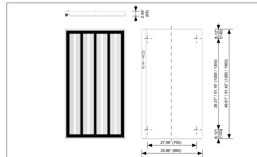
Außen- und Befestigungsmaße der LPS50 PM. Alle Angaben in Inch (mm).
