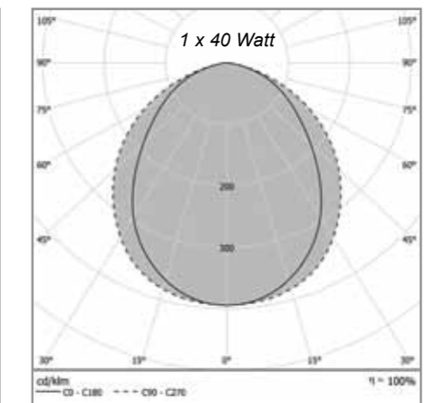
Lichtverteilungskurve der VAO PM (VAO puremaxLED®). Diese Grafik zeigt die Lichtverteilungskurve einer VAO PM mit 1 x 40 Watt
