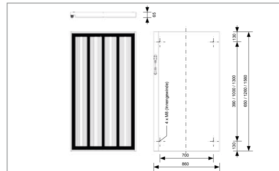
Außen- und Befestigungsmaße der LPS50 PM. Alle Angaben in mm.
