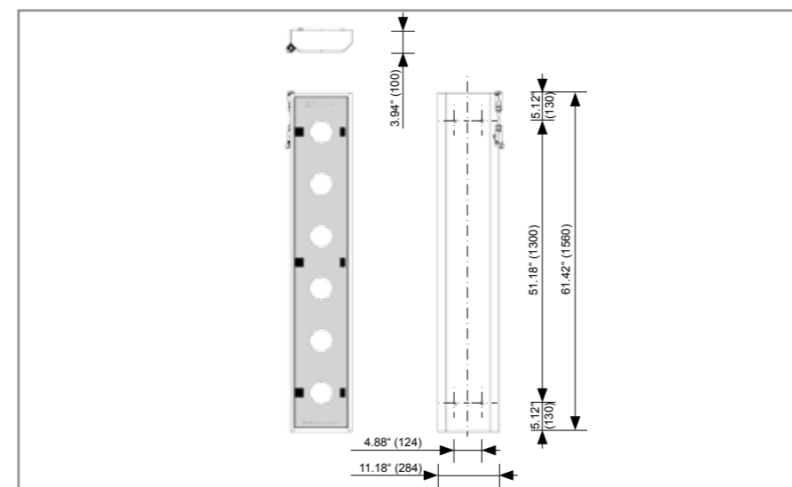
Außen- und Befestigungsmaße der LEDLPO. Alle Angaben in Inch (mm).
