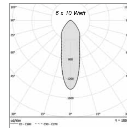
Lichtverteilungskurve der LEDLPO (LED-LightPointOptik). Diese Grafik zeigt die Lichtverteilungskurve einer LEDLPO mit 6 x 10 Watt.
