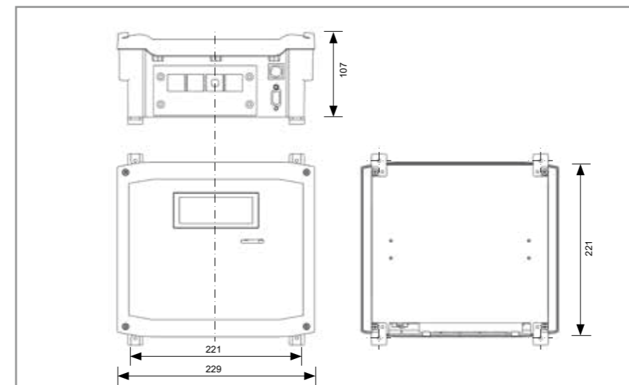
Außen- und Befestigungsmaße der HAST2.0. Alle Angaben in mm.
