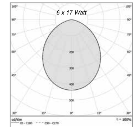
Lichtverteilungskurve der LEDSLO (LED-SunLightOptik). Diese Grafik zeigt die Lichtverteilungskurve einer LEDSLO mit 6 x 17 Watt.
