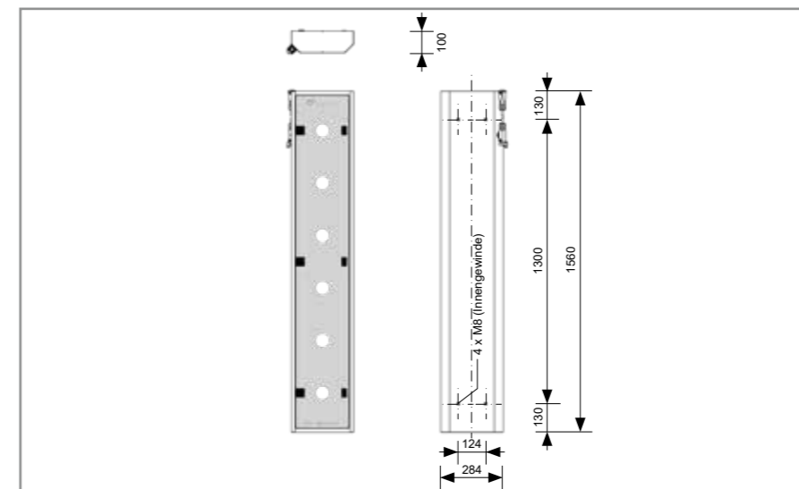
Außen- und Befestigungsmaße der LEDSLO. Alle Angaben in mm.
