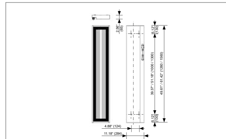
Außen- und Befestigungsmaße der VAO PM. Alle Angaben in Inch (mm).
