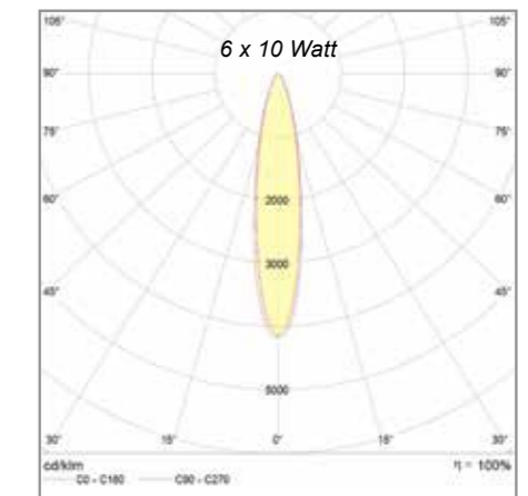
Lichtverteilungskurve der LEDLPO (LED-LightPointOptik). Diese Grafik zeigt die Lichtverteilungskurve einer LEDLPO mit 6 x 10 Watt.
