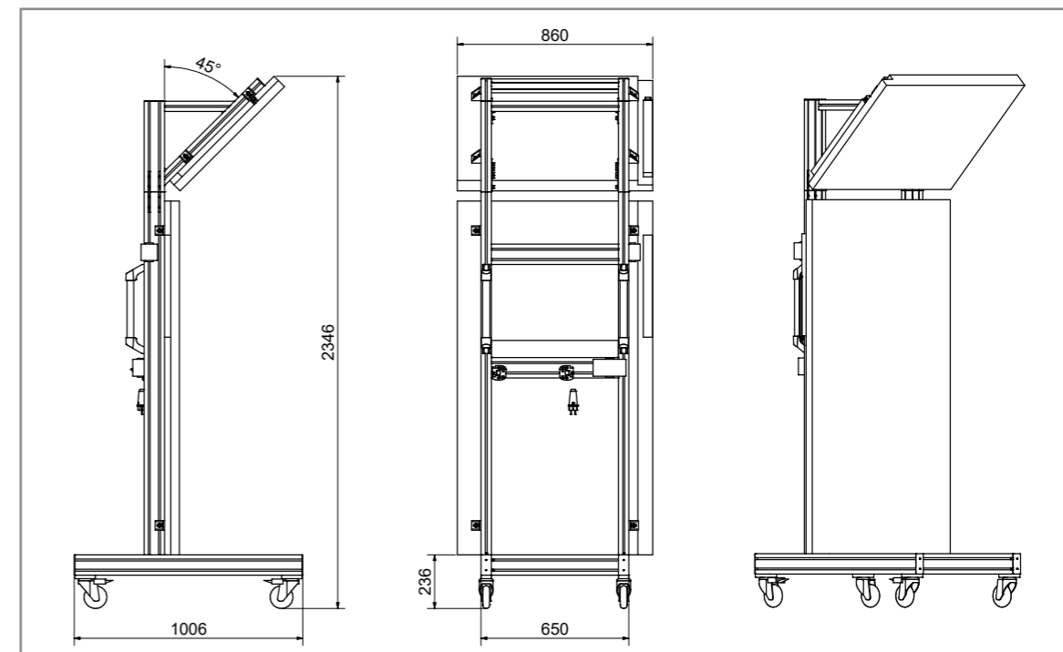
Außenmaße der mobilen Prüfstation LPS100 PM (5ft. & 2ft.). Alle Angaben in mm.
